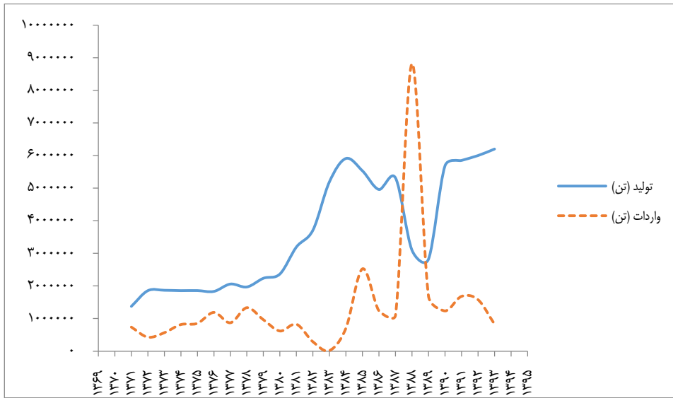
نمودار ۱- روند تولید و واردات شکر ایران در سال‌های ۹۳-۱۳۷۱
